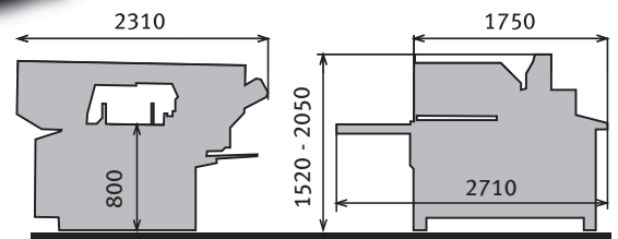
Fig. : BMBS 300 x 320 CNC-G
